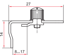
УПЗ-2 (нерж.)
