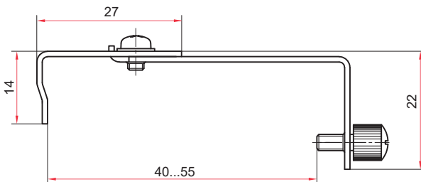
УПЗ-5 (нерж.)
