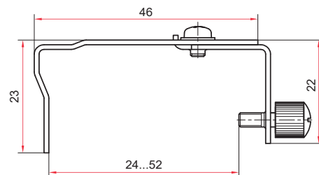
УПЗ-1 (нерж.)
